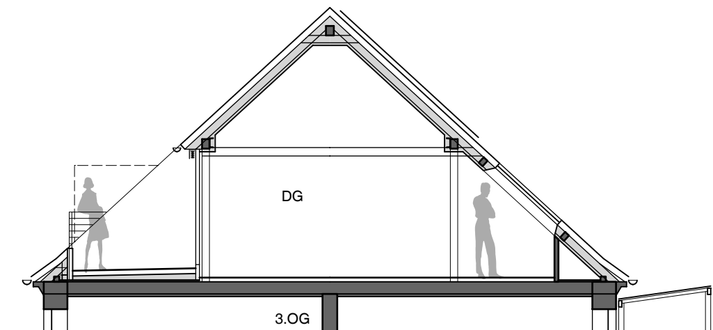
Schnitt Dachterrasse
