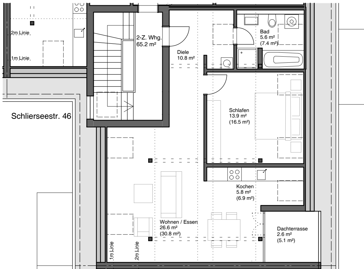
Grundriss
