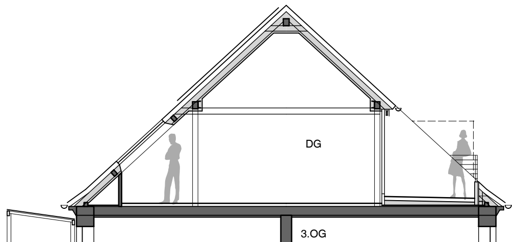
Schnitt Dachterrasse
